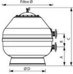
Astralpool Volcano Havuz Kum Filtresi Ölçü Tablosu
